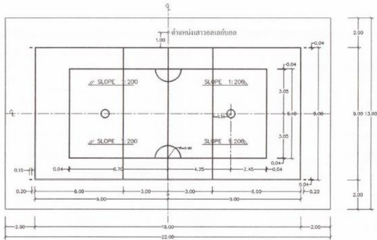
แปลนสนาม มาตราส่วน 1 : 100
