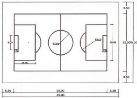
แปลนสนามฟุตบอล 7 คน แบบไม่ปูหญ้า มาตราส่วน 1 : 500
